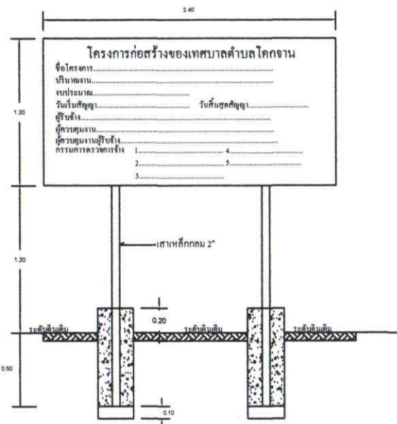
แบบป้ายโครงการ
